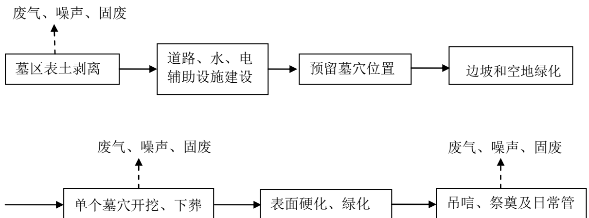
图 3-4 生产工艺流程图及产污环节
