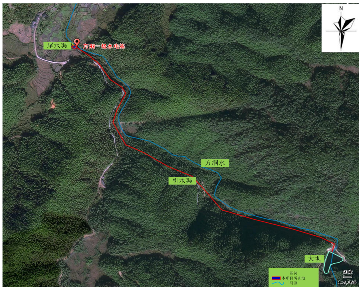
附图3 本项目引水、排水工程示意图
