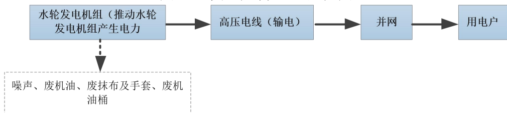
图 2-2 升压站工艺流程图
