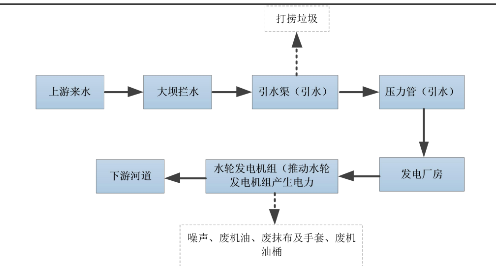
图 2-1 发电厂房工艺流程图
