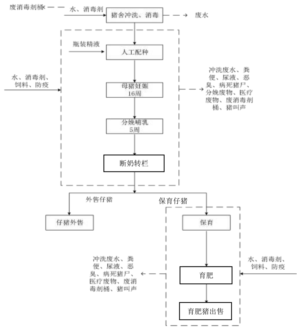
图 3-9 本项目主要生产工艺流程图
