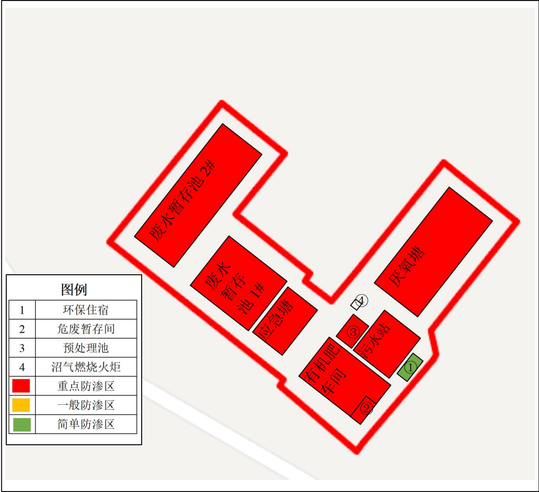
图 6-5 项目环保区地下水分区防渗示意图
