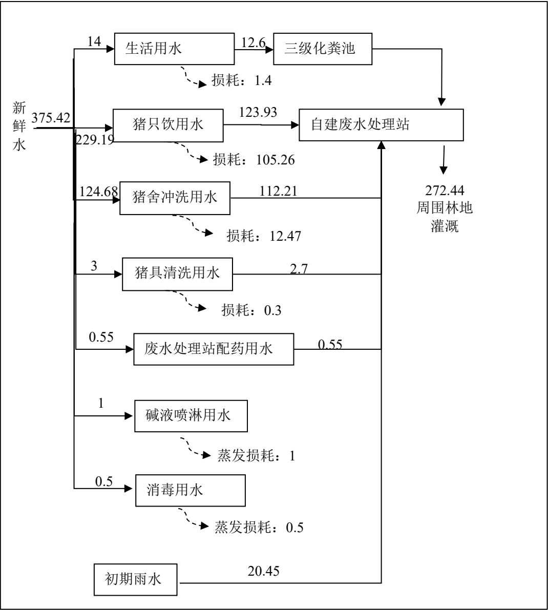
图 3-6 本项目非雨季水平衡示意图（单位 \text{m}^3/\text{d} ）
