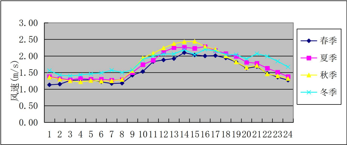
图5-4 始兴气象站2022年季小时平均风速的日变化图
