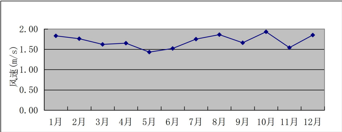
图5-3 始兴气象站2022年各月平均风速变化图
