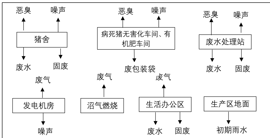
图 3-16 项目产污节点图
