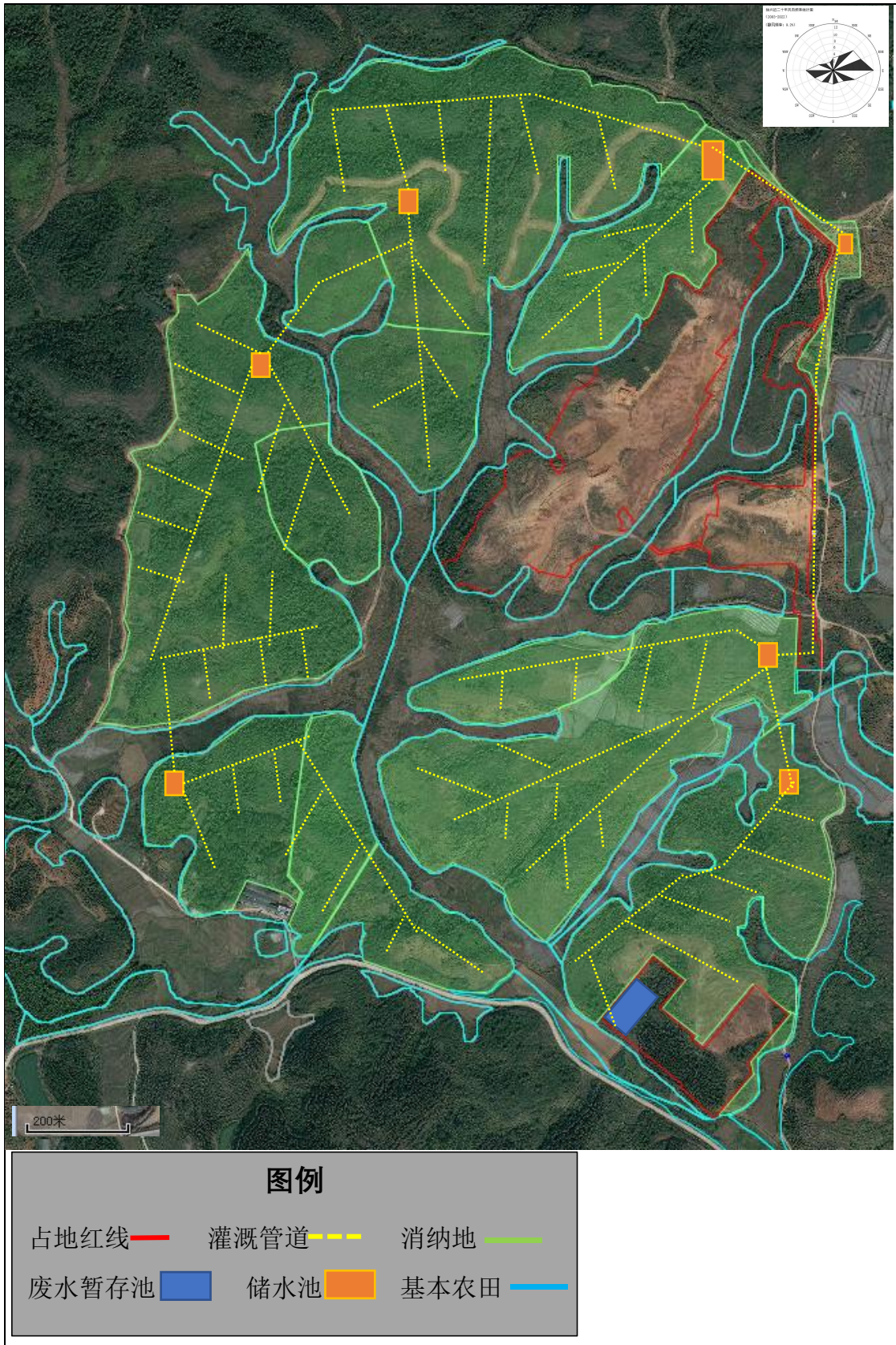
图 6-3 灌溉管网布置示意图
