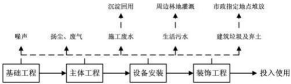
图 3-8 施工期工艺流程及产污节点图
