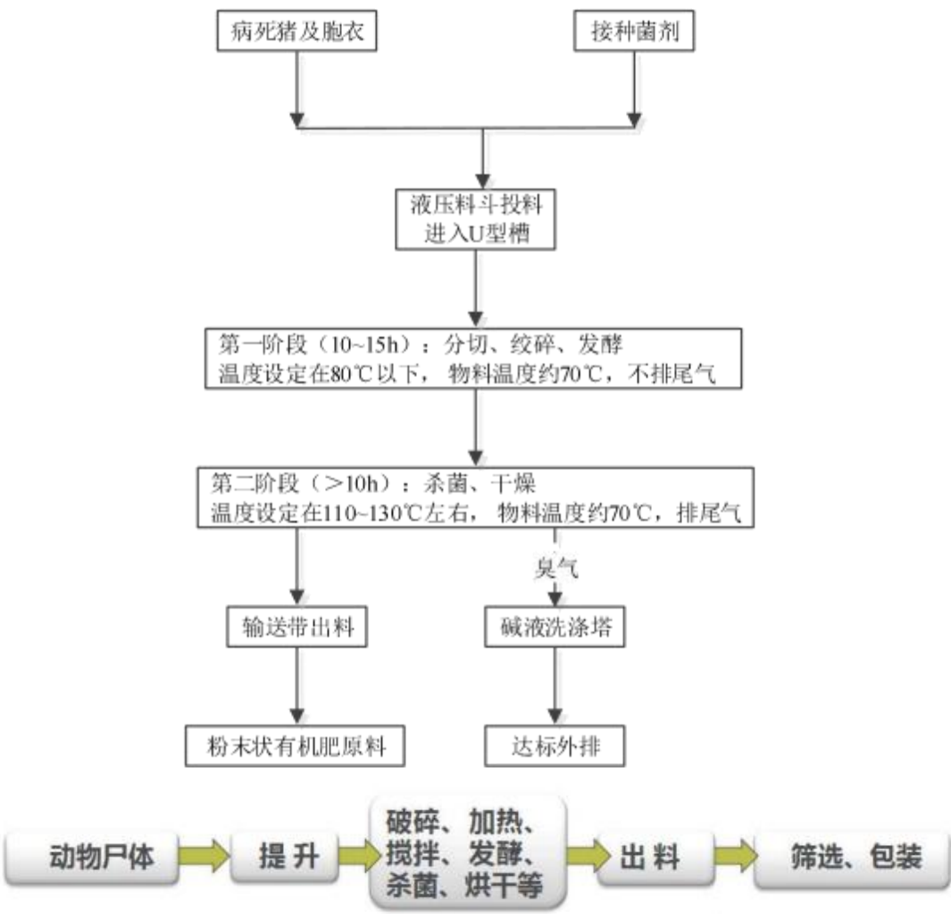
图 3-14 病死猪和分娩物制肥工艺流程
