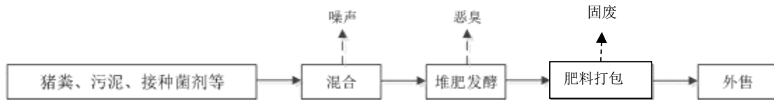
图 3-13 有机肥生产工艺流程
