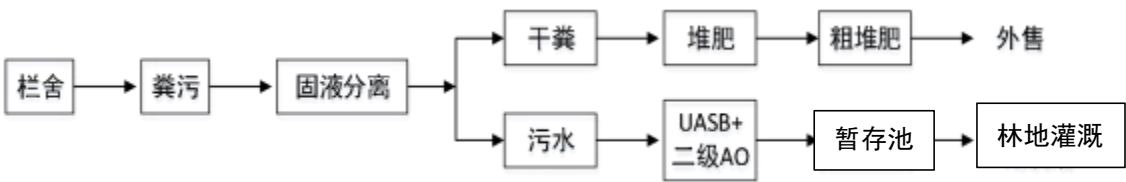
图 3-11 粪污处理工艺示意图
