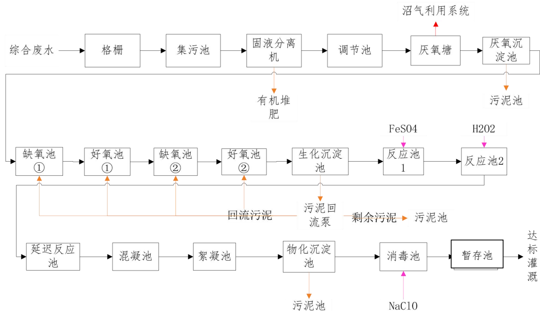
图6-2 废水处理工艺流程图
