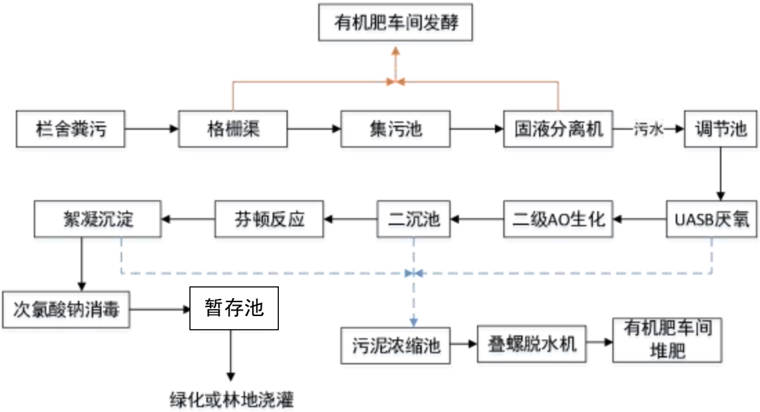
图3-17 污水处理站工艺流程
