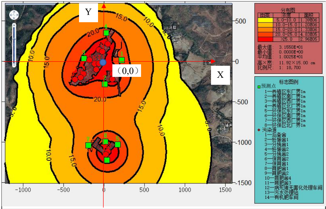
图 5-29 声环境预测坐标体系及等声级线图
