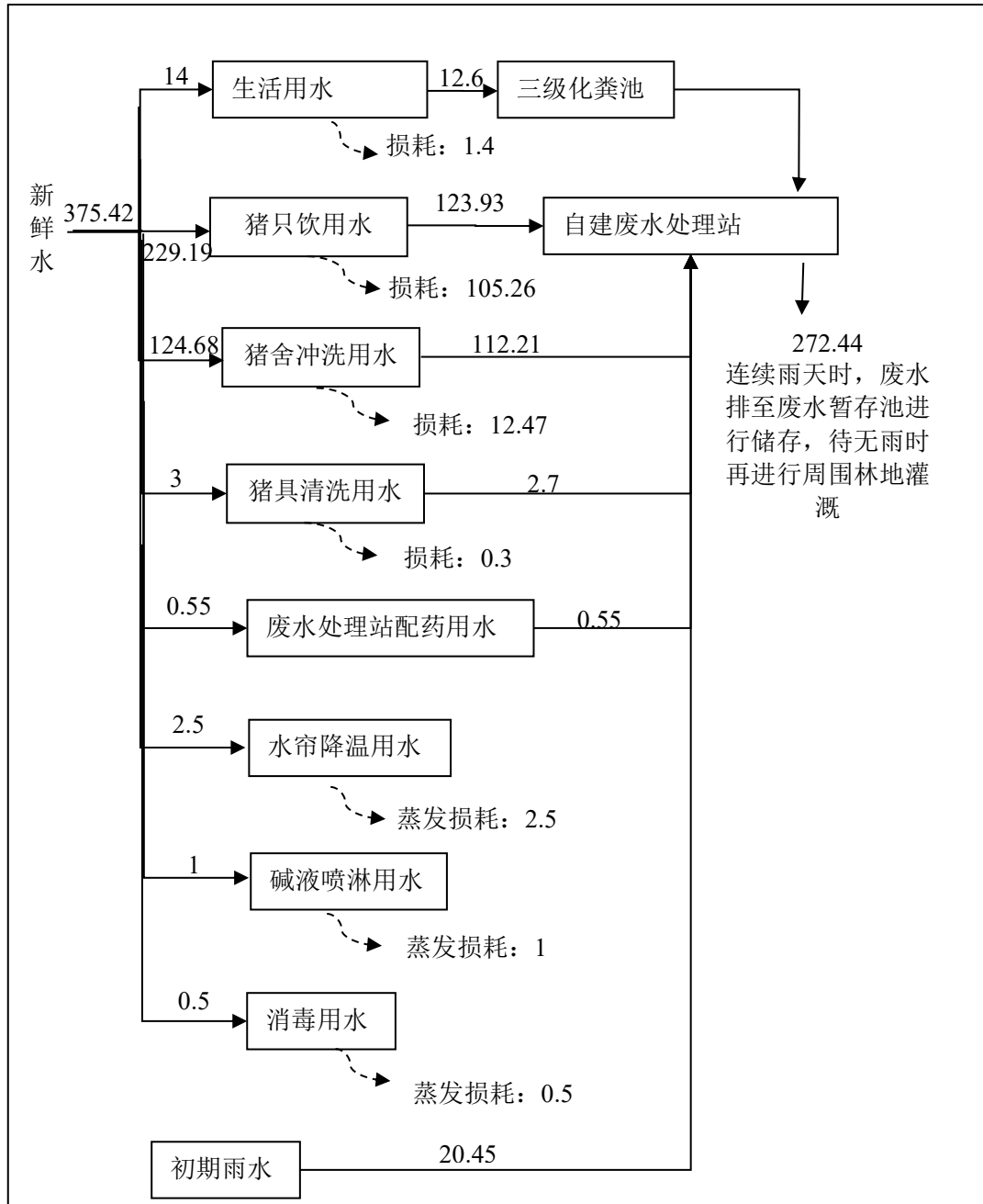
图 3-7 本项目雨季水平衡示意图 (单位 \text{m}^3/\text{d} )
