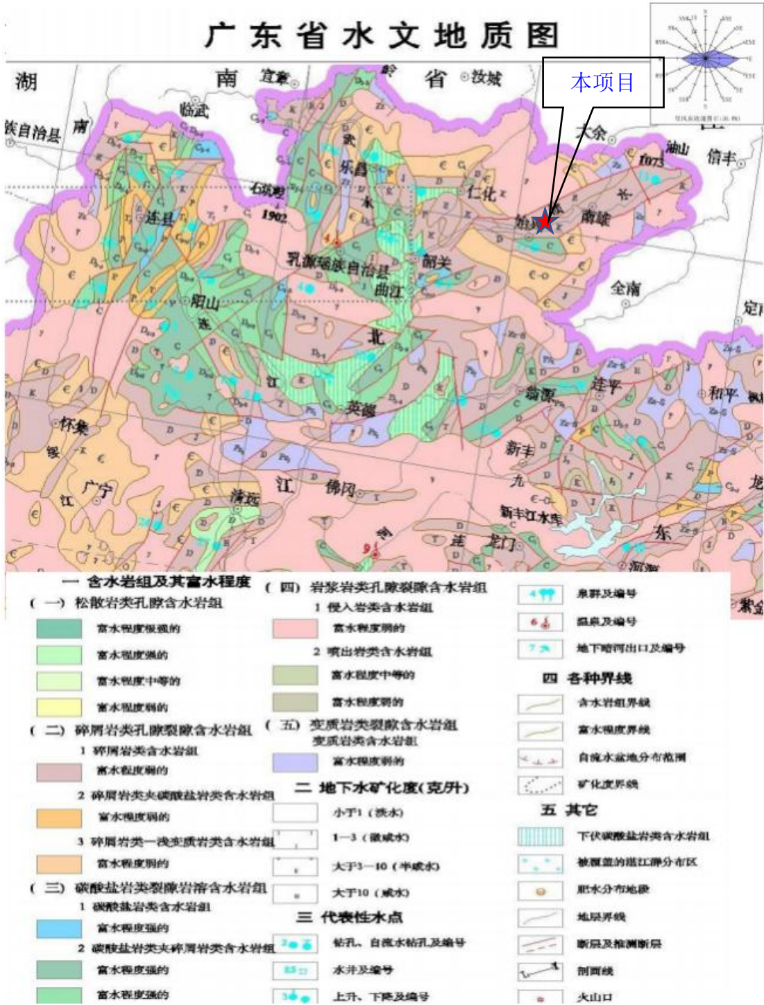
图 5-27 项目所在区域水文地质状况图
