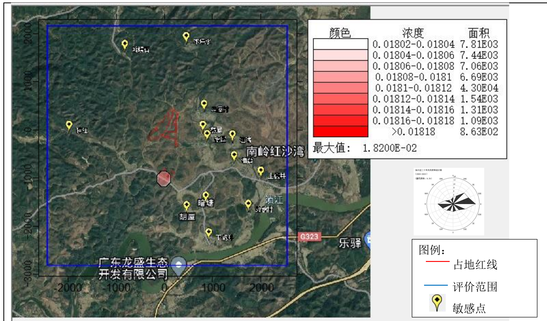
图 5-22 正常排放 \text{NO}_2 年平均浓度叠加值分布图 ( \text{mg}/\text{m}^3 )
