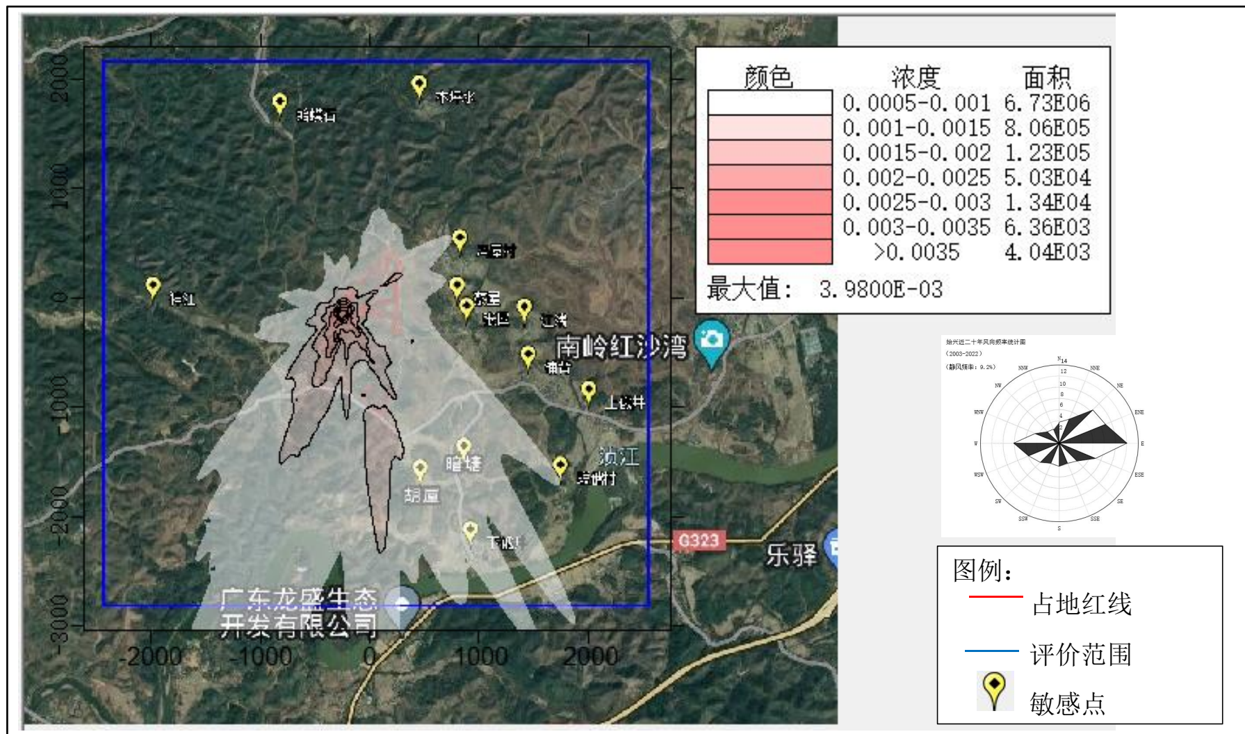
图 5-18 正常排放 H_2S 一小时平均浓度叠加值分布图 ( mg/m^3 )
