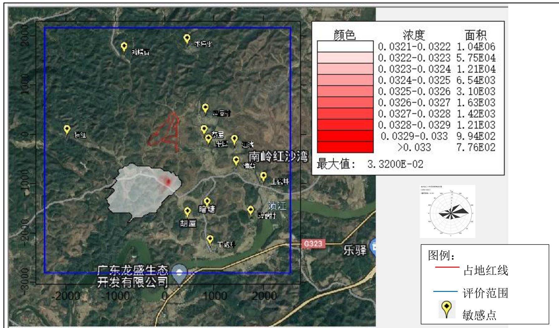
图 5-21 正常排放 \text{NO}_2 日平均 (98%保证率) 浓度叠加值分布图 ( \text{mg}/\text{m}^3 )
