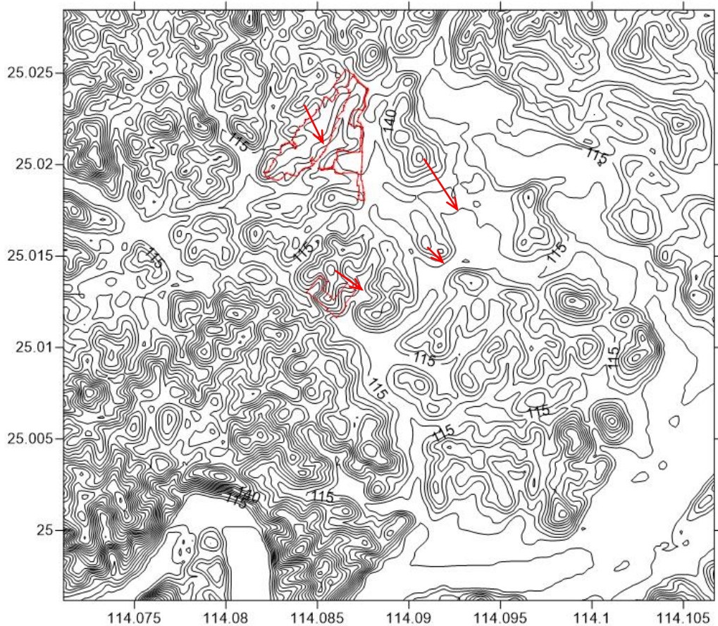
图 5-28 项目地下水流向图
