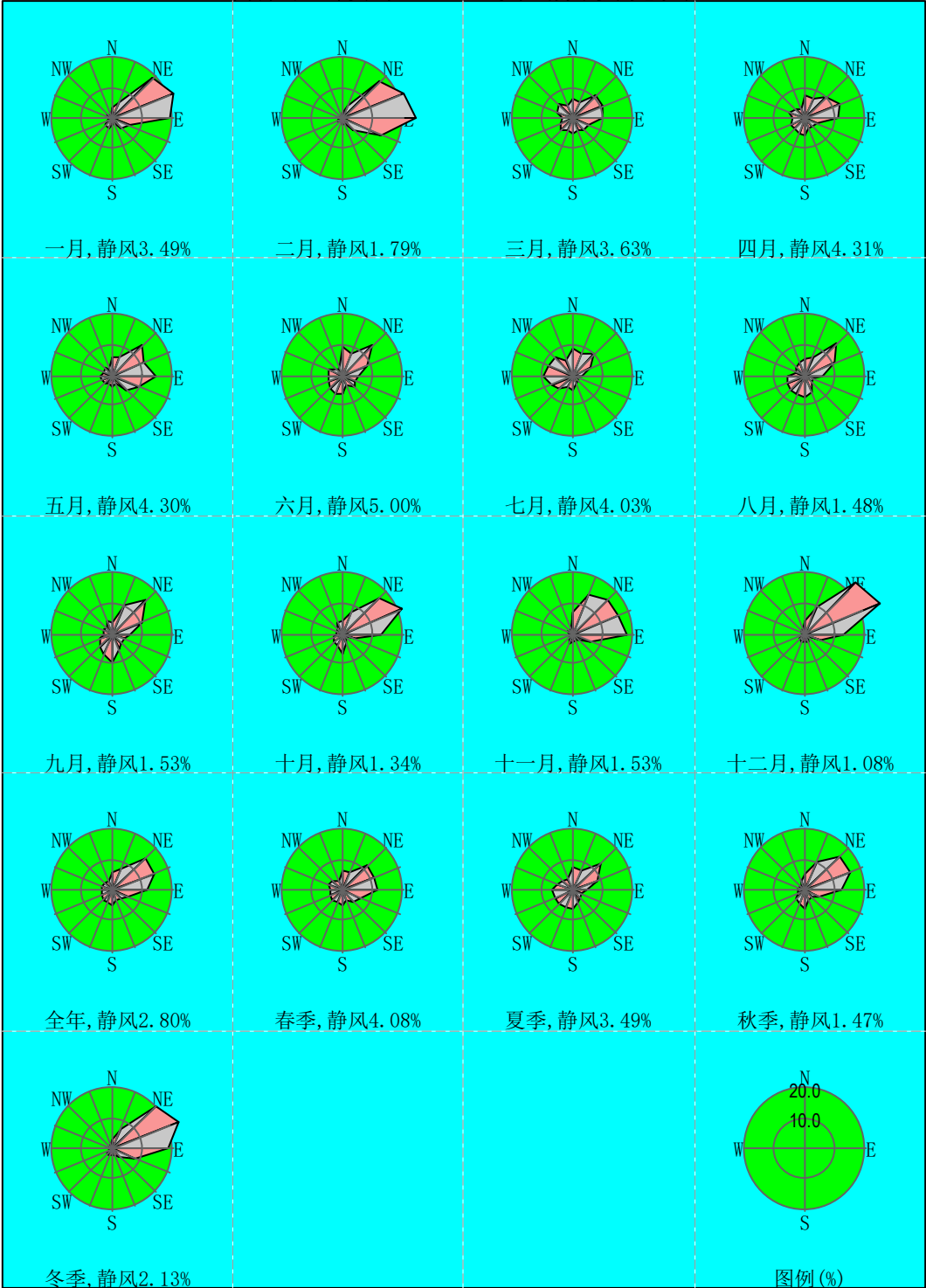
图 5-5 始兴气象站 2022 年四季和全年风向玫瑰图
