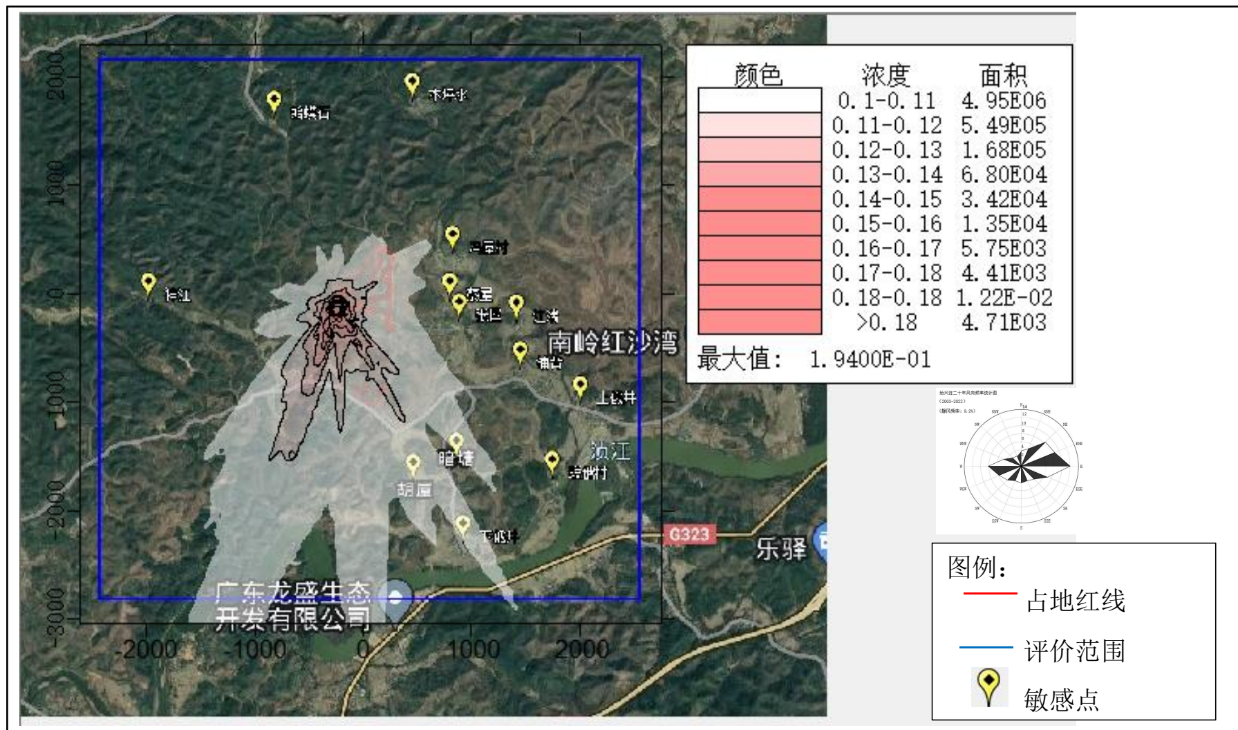
图 5-17 正常排放 \text{NH}_3 一小时平均浓度叠加值分布图 ( \text{mg}/\text{m}^3 )
