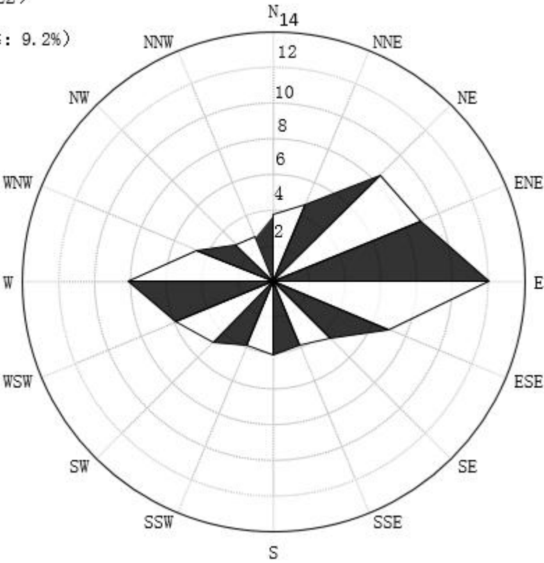
始兴近二十年风向频率统计图 (2003-2022)
