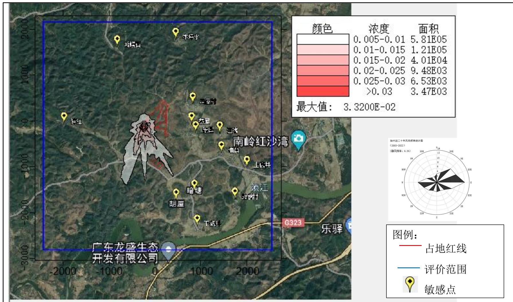
图 5-26 非正常排放 H_2S 小时浓度贡献值分布图 ( mg/m^3 )
