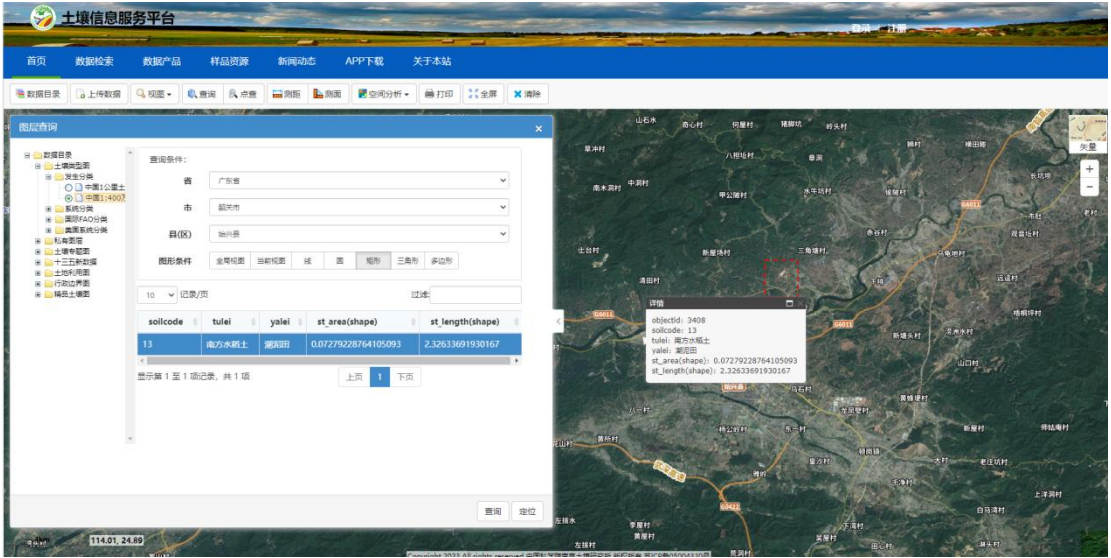
图4-2 土壤类型图
