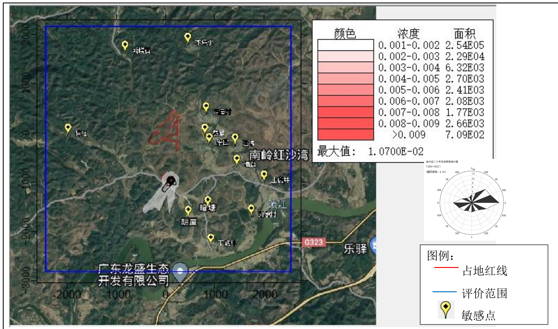
图 5-12 正常排放 \text{NO}_2 一小时平均浓度各点贡献高值分布图 ( \text{mg}/\text{m}^3 )
