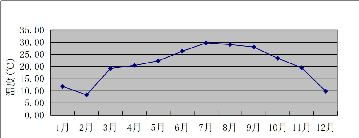
图5-2 始兴气象站2022年平均温度的月变化图
