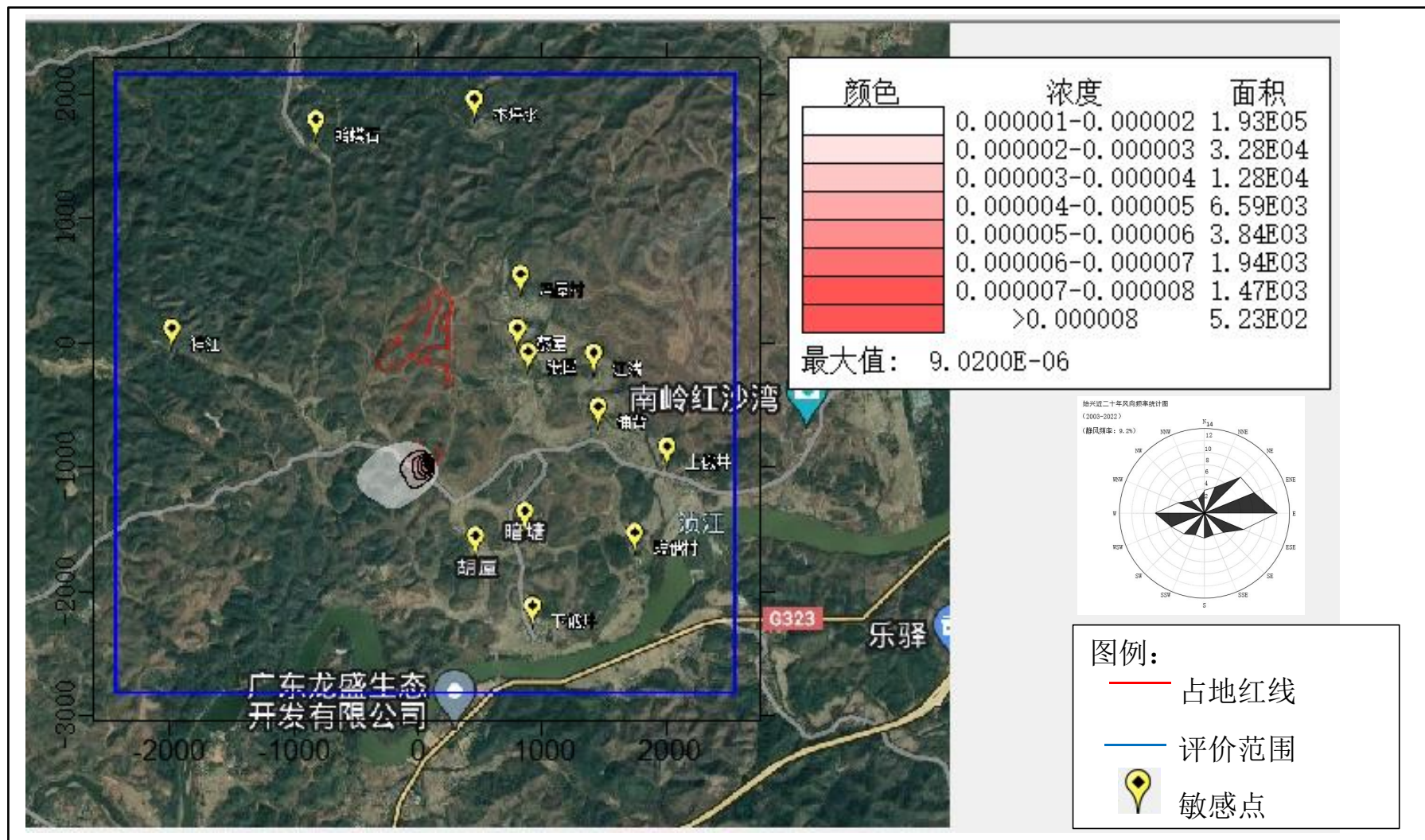
图 5-11 正常排放 SO 2 年均浓度各点贡献高值分布图 (mg/m 3 )
