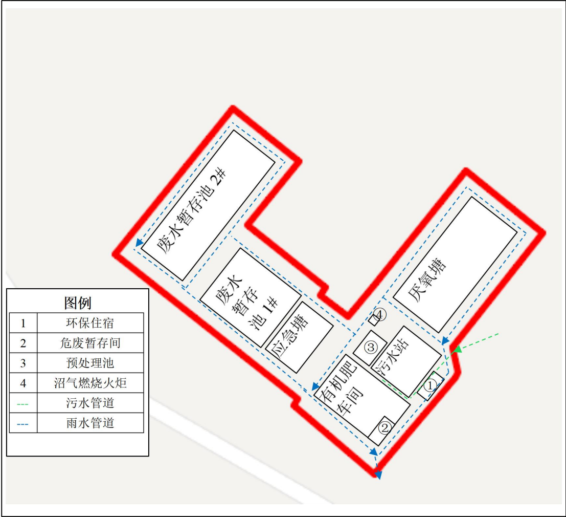
图 3-5 项目环保区平面布置及雨污管网
