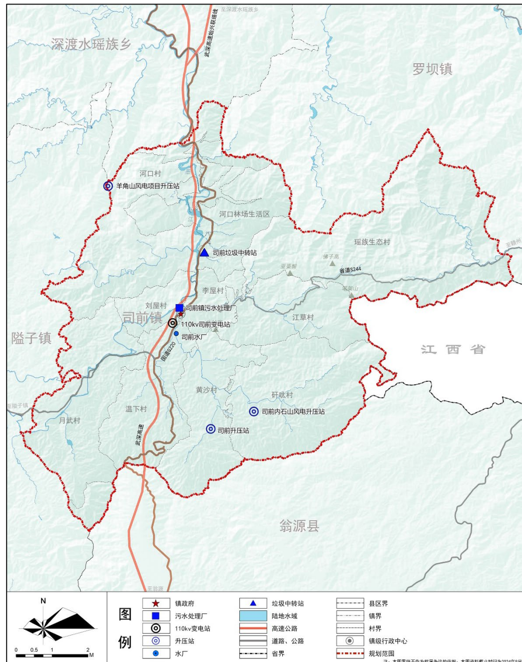
镇域重大基础设施规划图
