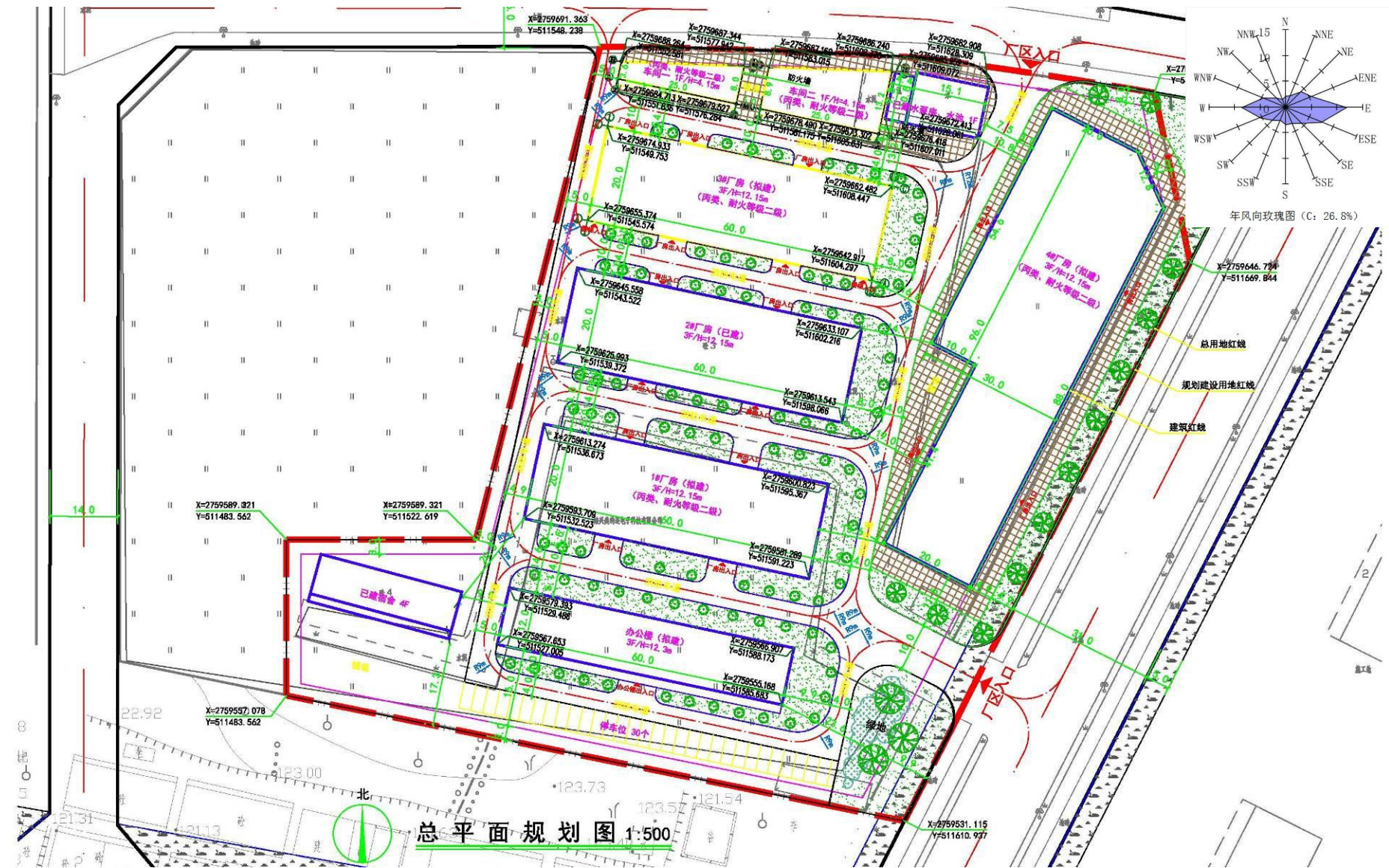
附图 7：项目厂区总平面规划图
