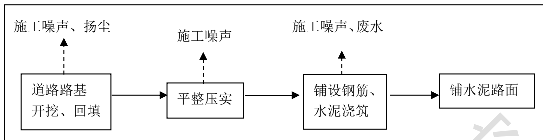
图7 道路施工工艺流程及产污节点图
