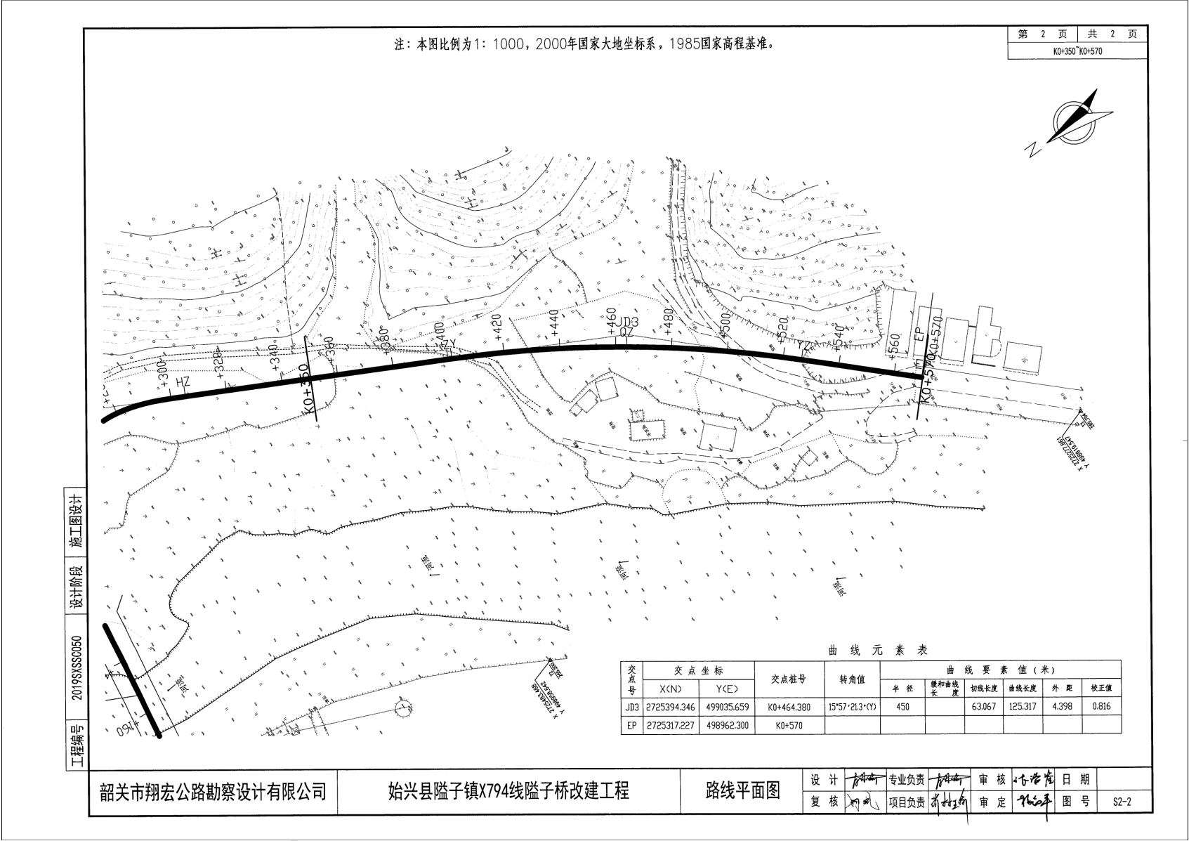
图 2 路线平面图（二）
