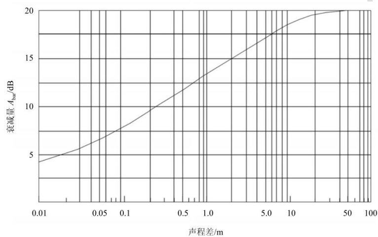
图 15 噪声衰减量 A_{\text{bar}} 与声程差 \delta 关系曲线 ( f=500 \text{ Hz} )
