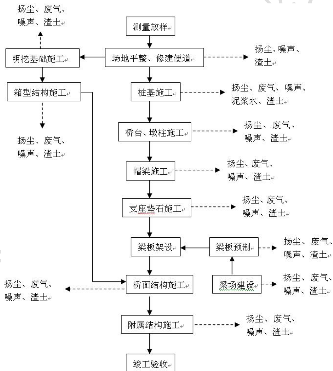
图8 桥梁施工工艺流程及产污节点图
