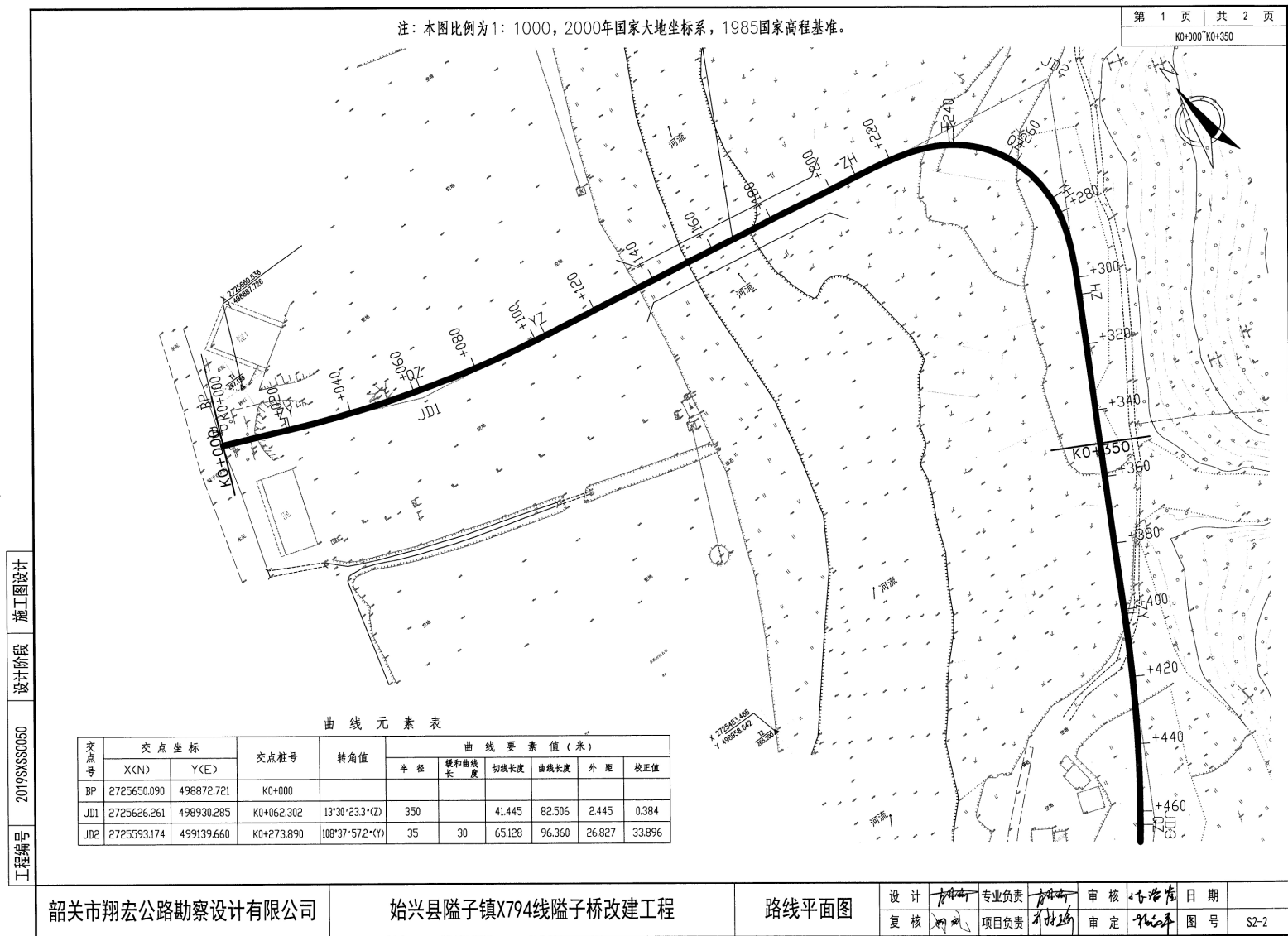
图 2 路线平面图（一）
