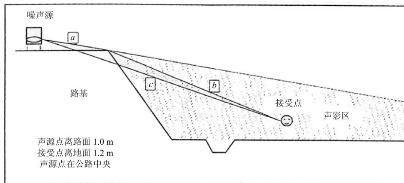
图 14 声程差 \delta 计算示意图
