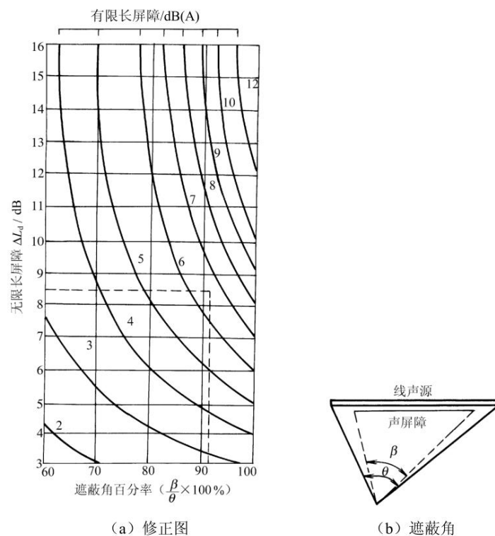
图 11 有限长度的声屏障及线声源的修正图
