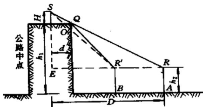
图 12 高路堤声照区及声影区示意图
