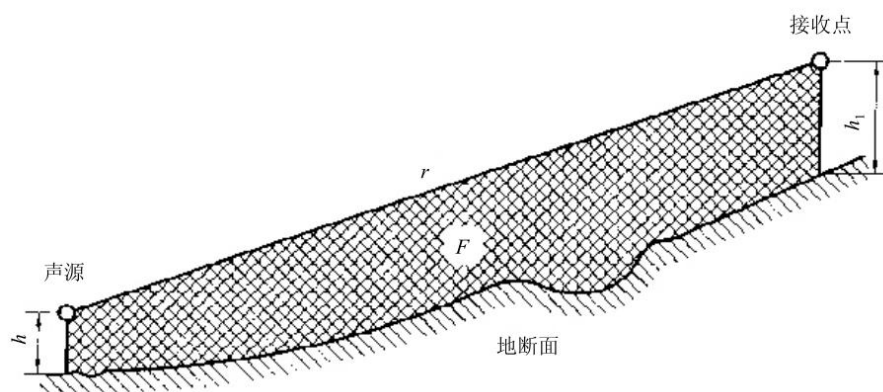
图 18 估计平均高度 h_m 的方法
