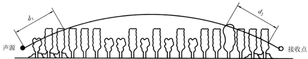
图 17 通过树和灌木时噪声衰减示意图
