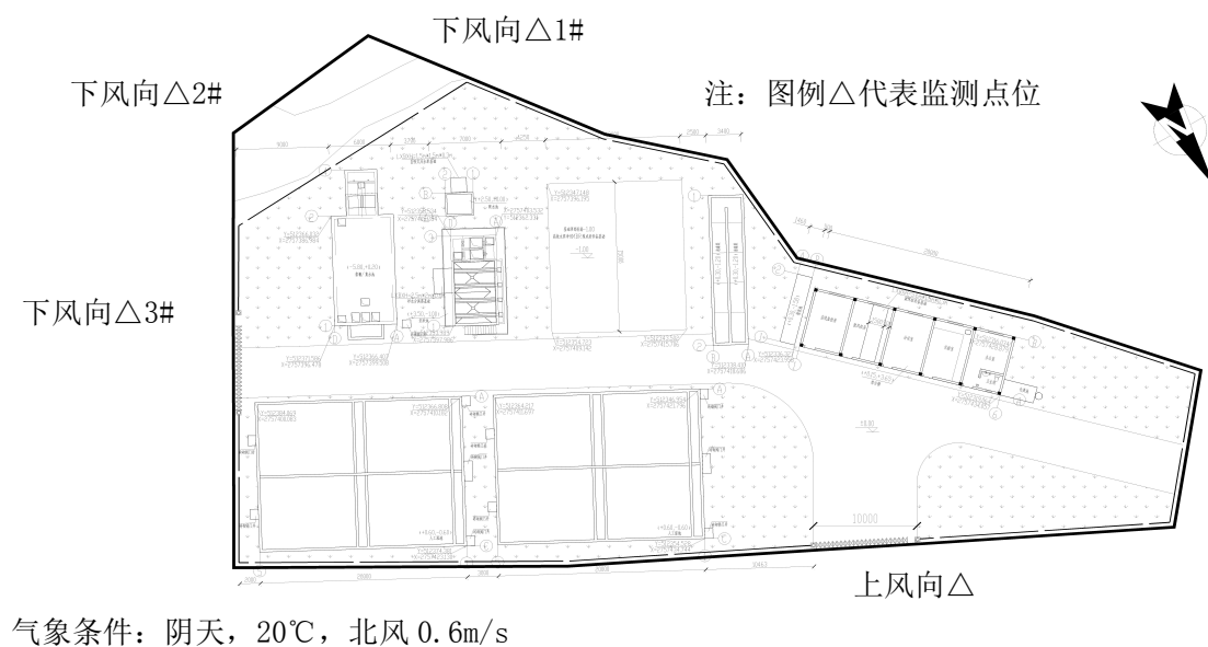
图 7-1 无组织废气监测点位布置图
